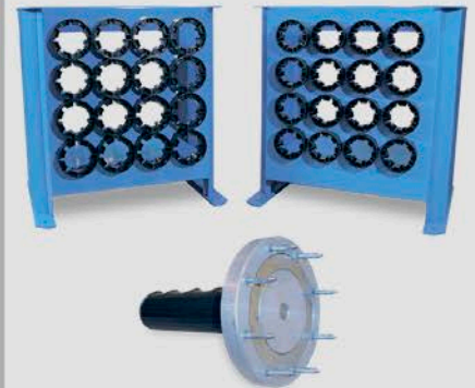
Инструментальная база и рамка для кулачков с устройством быстрой замены
